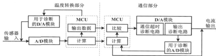
图 2 安全温度变送器诊断逻辑图
