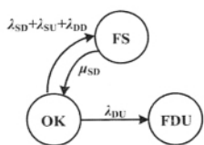
图 3 Markov 状态转移图
