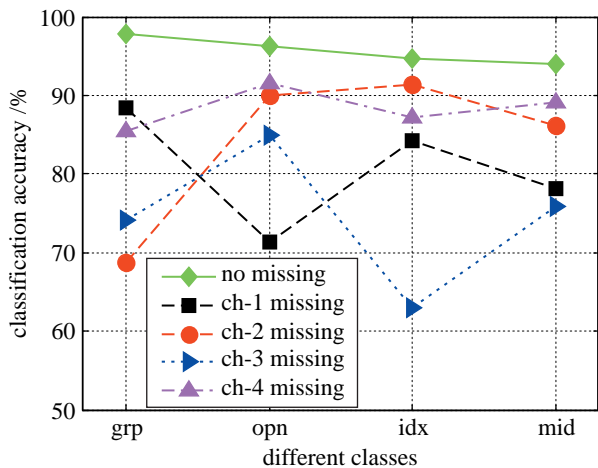
图 7 不同通道数据丢失条件下计算的分类精度
