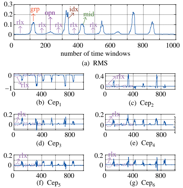
图 5 由图 2 中第 3 通道 sEMG 数据提取的特征，其中 rlx 占有超过 50% 的数据。(a) 均方根；(b) ~ (g) 倒谱系数
