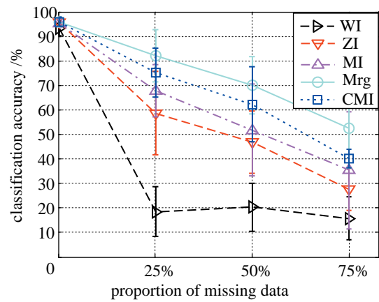
图 6 识别除 rlx 外 4 种手部动作时不同方法计算的分类精度均值和标准差 (WI 直接使用错误值, ZI 零归错, MI 均值归错, Mrg 边缘化, CMI 条件均值归错; 25%: 1 个通道, 50%: 2 个通道, 75%: 3 个通道)
