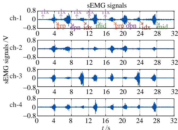
图 2 一组试验的原始表面肌电信号 Fig.2 The raw sEMG signals in an experiment session
