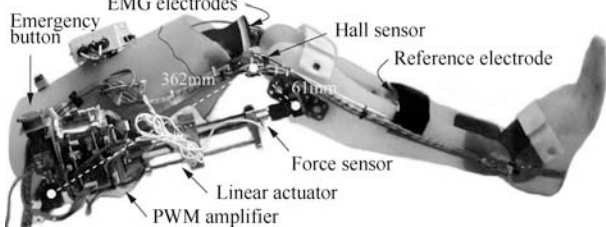
图 11 TUPLEE 下肢外骨骼 Fig. 11 The TUPLEE lower extremity exoskeleton
