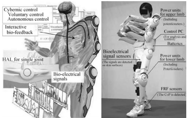
图 12 HAL 外骨骼 Fig. 12 The HAL exoskeleton
