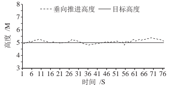
图 7 两种推进方式下的深/高度对比 Fig.7 Height/depth comparison under the two propulsion control
