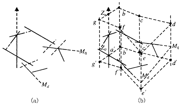
图2 操作手始末位姿及工作空间
