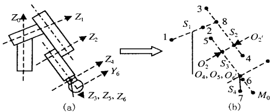
图1 机械手手臂细化
