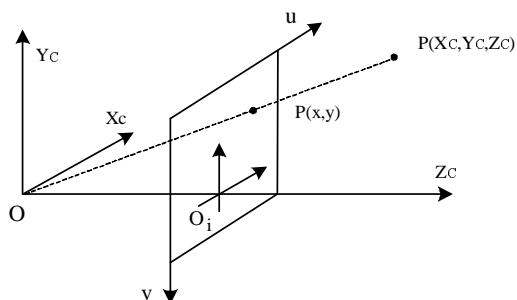
图1 小孔成像模型
