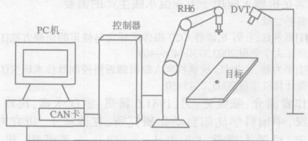
图2 系统结构示意图
